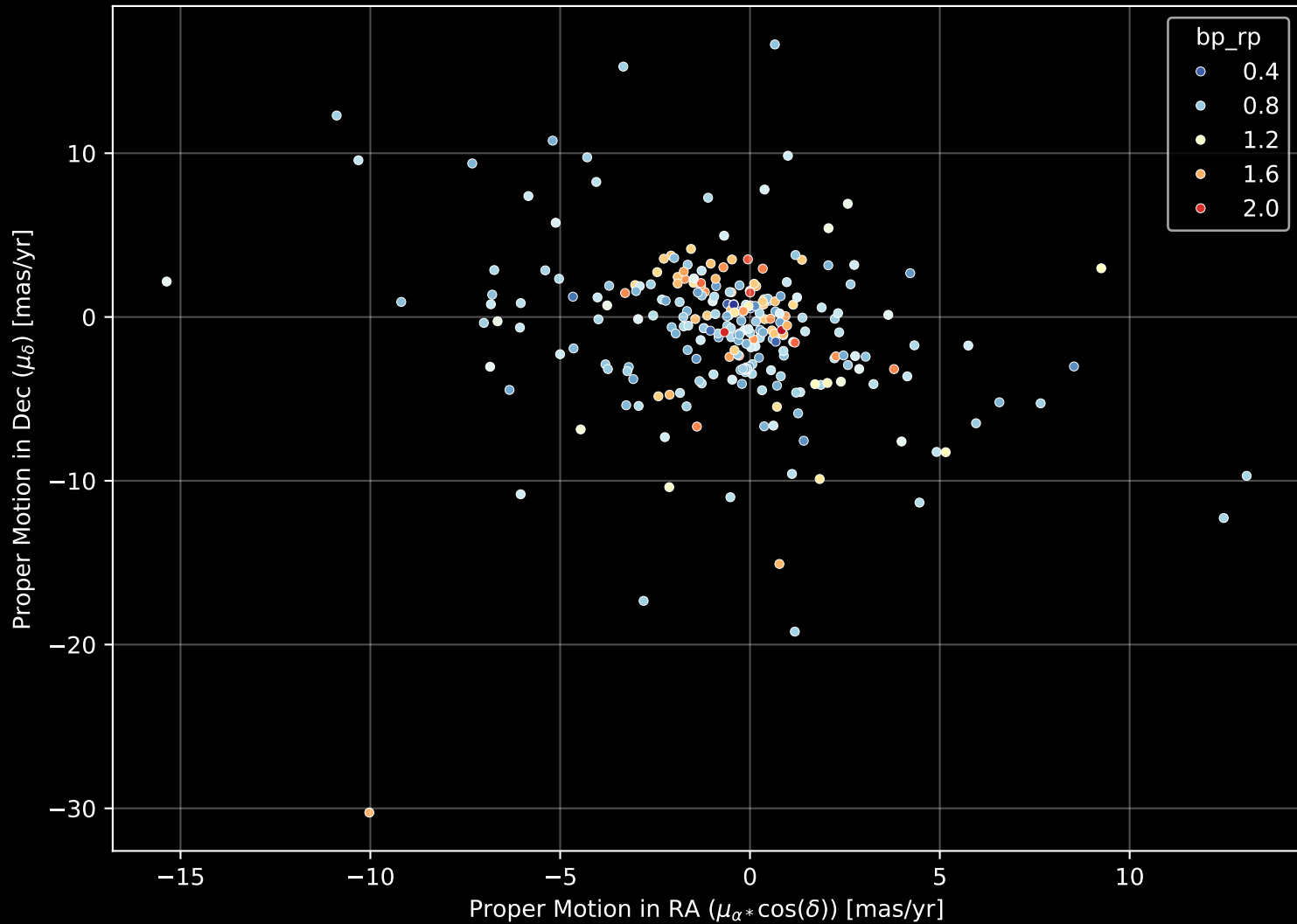
GALAH DR4 Field: [9028] Proper Motion Diagram (n= 262)
