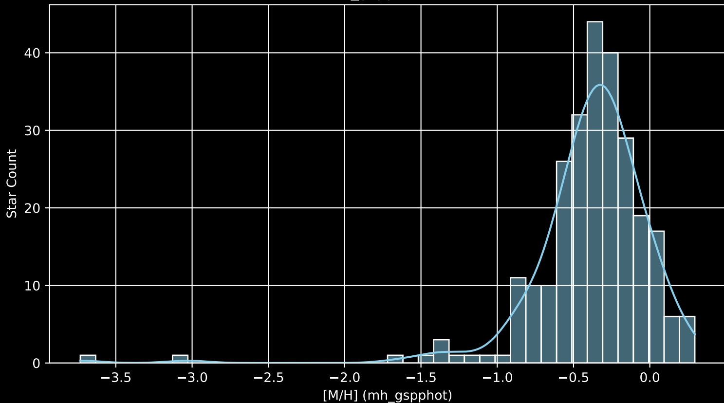
GALAH DR4 Field: [9028] [M/H] (mh_gspphot) (n= 261)
