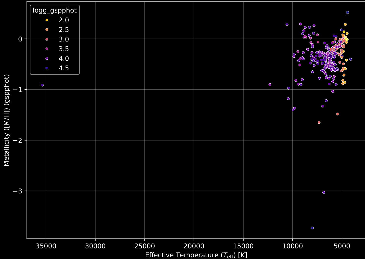
GALAH DR4 Field: [9028] Stellar Population Parameters (n= 262)
