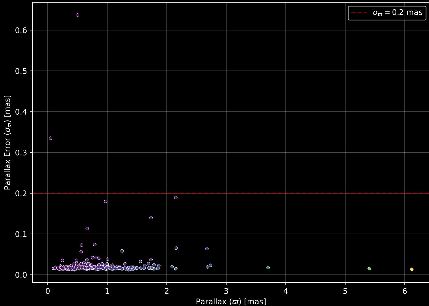
GALAH DR4 Field: [9028] Parallax Quality (n= 262)
